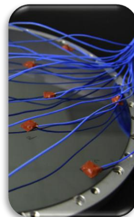
E-Chuck 靜電卡盤 Heater 加熱器 Electrode 電極
